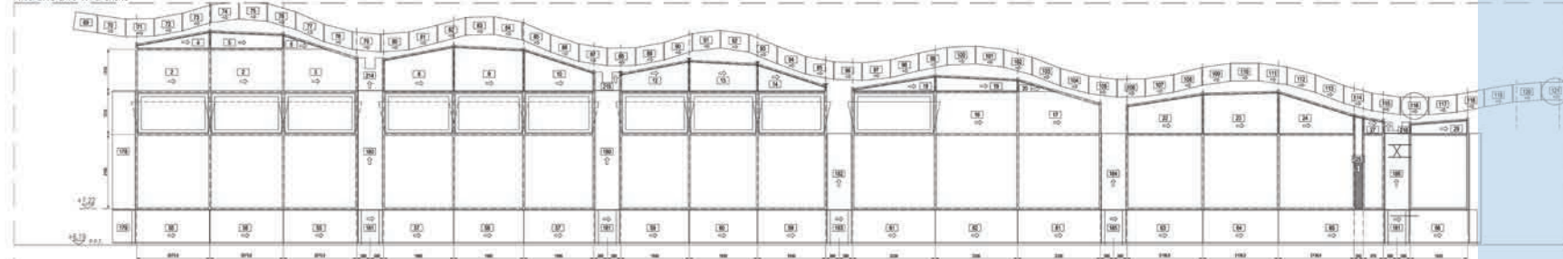
PROSPETTO LATO VIA G. BRUNO
